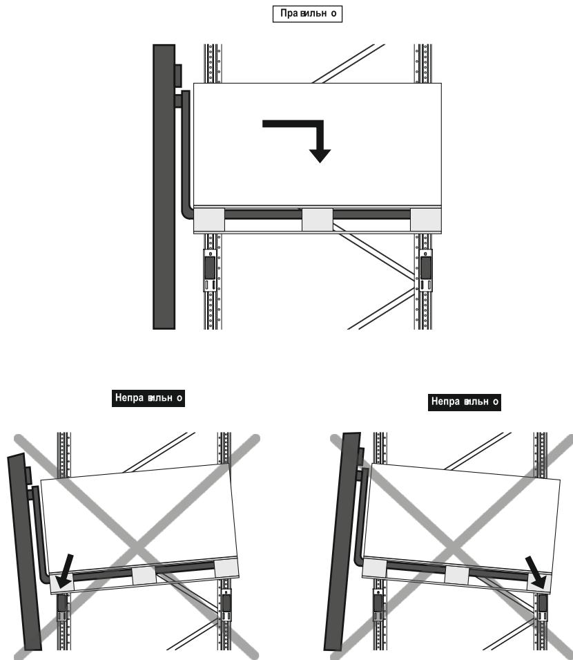
Рисунок 18 - Установка грузовой единицы на балки
