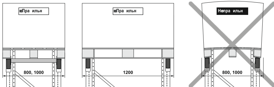
Рисунок 4 - Расположение грузовой единицы на балках
