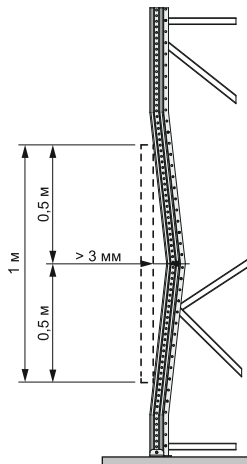
Рисунок 20 - Виды повреждений стойки
